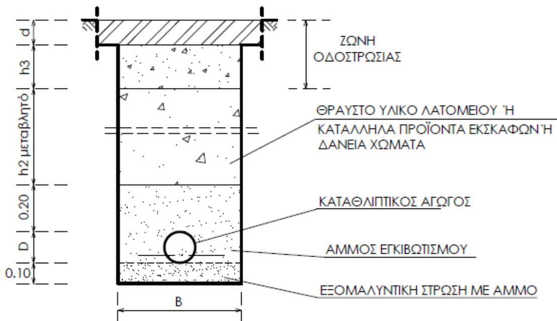
Σχήμα Π10: Τυπικό σκάμμα τοποθέτησης καταθλιπτικού αγωγού.
