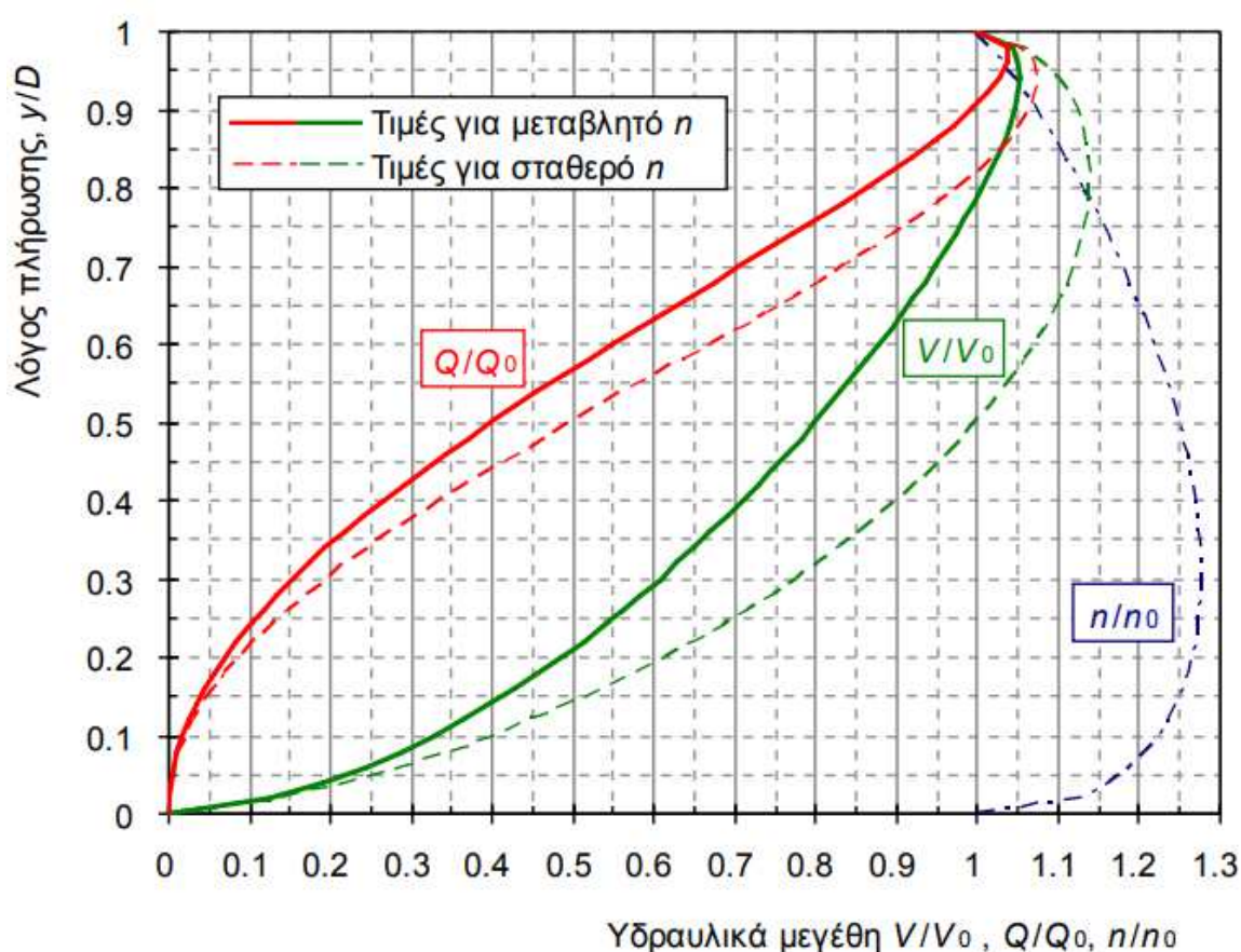
Σχήμα Π4: Μεταβολή των υδραυλικών μεγεθών ροής με ελεύθερη επιφάνεια σε κυκλικούς αγωγούς συναρτήσει του λόγου πλήρωσης y/D .
