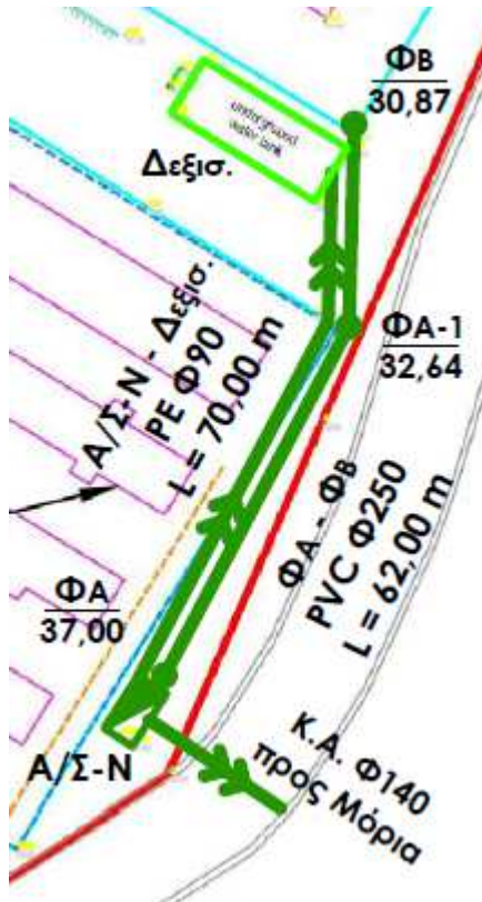
Σχήμα 1: Διάταξη του αποχετευτικού δικτύου στο εσωτερικό του ΚΥΤ (Πηγή: μελέτη [1]).
