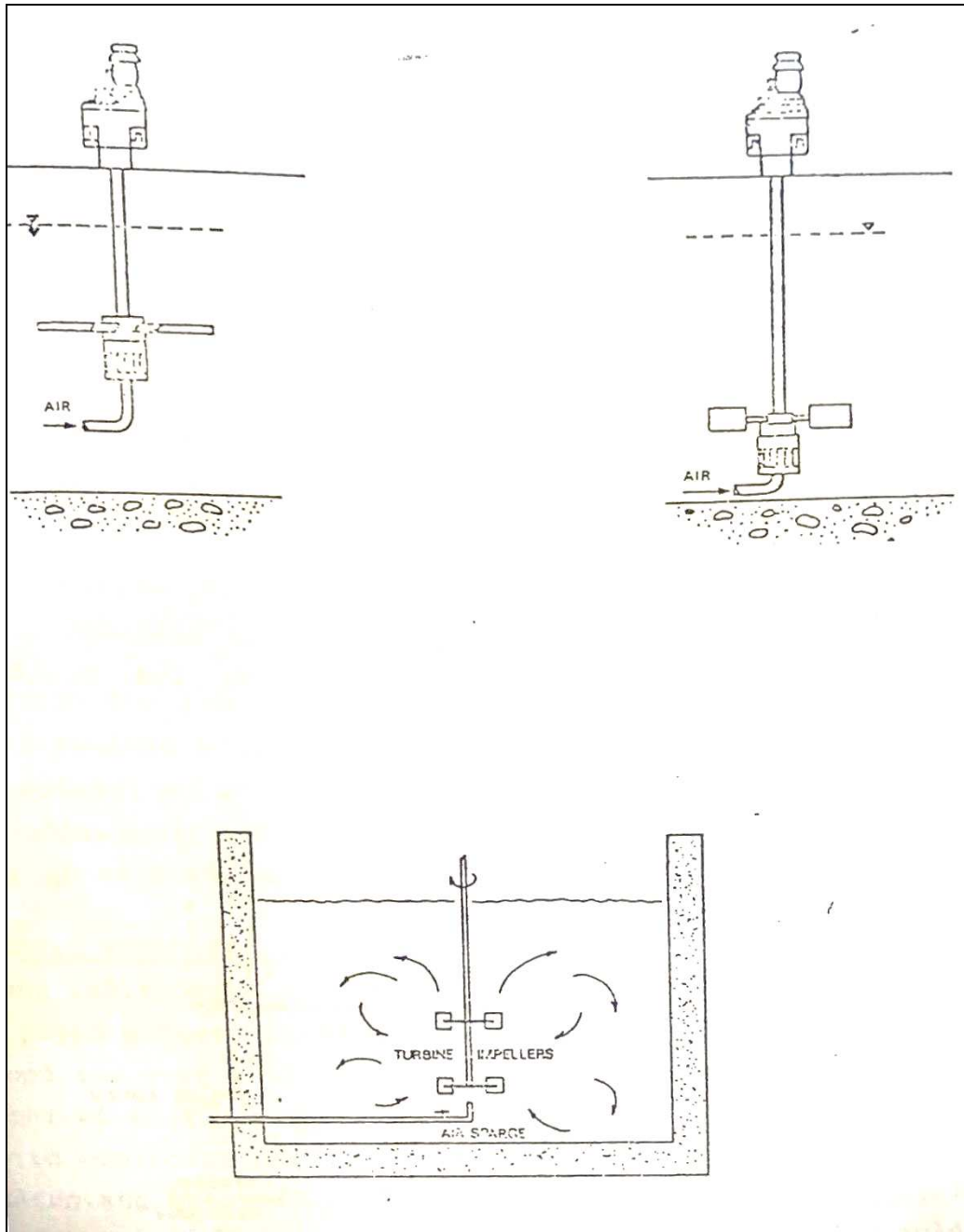
Σχήμα 4: Τυπικά συστήματα βυθισμένων αεριστών με στρόβιλο 1 .
