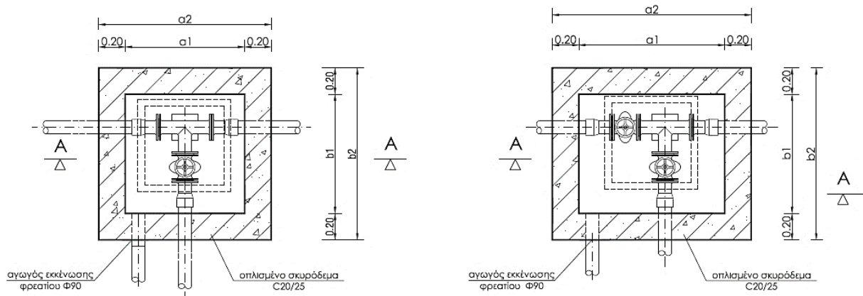
Σχήμα Π6: Κάτοψη φρεατίων δικλείδων από σκυρόδεμα.
