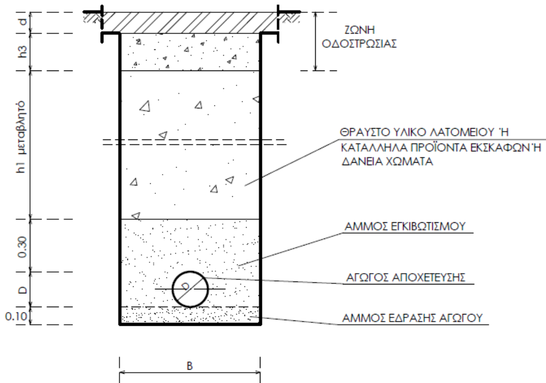
Σχήμα Π9: Τυπικό σκάμμα τοποθέτησης αγωγού βαρύτητας.
