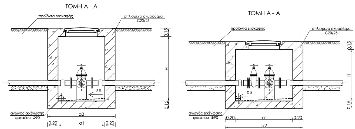
Σχήμα Π7: Τομή φρεατίων δικλείδων από σκυρόδεμα.
