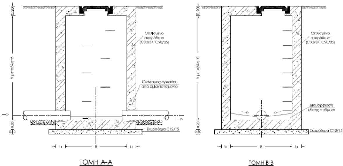
Σχήμα Π8: Τομή φρεατίων επίσκεψης αγωγών ελεύθερης ροής από σκυρόδεμα.
