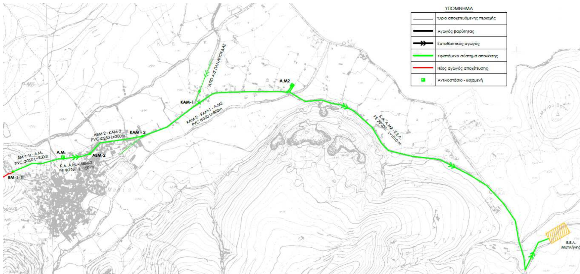
Σχήμα Π2: Γενική διάταξη του υφιστάμενου συστήματος αγωγών μεταφοράς λυμάτων στην ΕΕΛ (Πηγή: μελέτη [1]).
