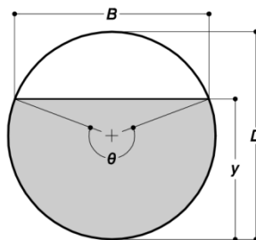
Σχήμα Π3: Γεωμετρία ροής σε αγωγό κυκλικής διατομής με μερική πλήρωση.
