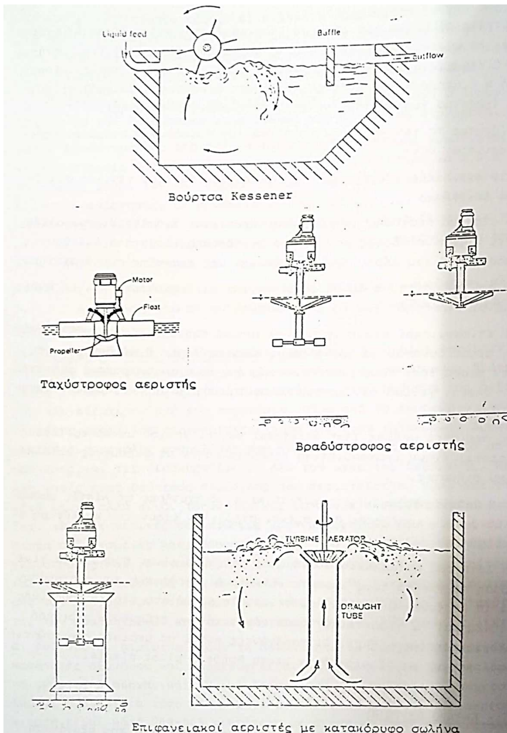
Σχήμα 3: Τυπικοί επιφανειακοί αεριστές 1 .
