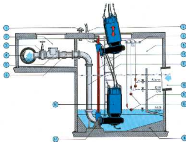
Σχήμα 6: Παράδειγμα υποβρύχιας εγκατάστασης αντλίας.
