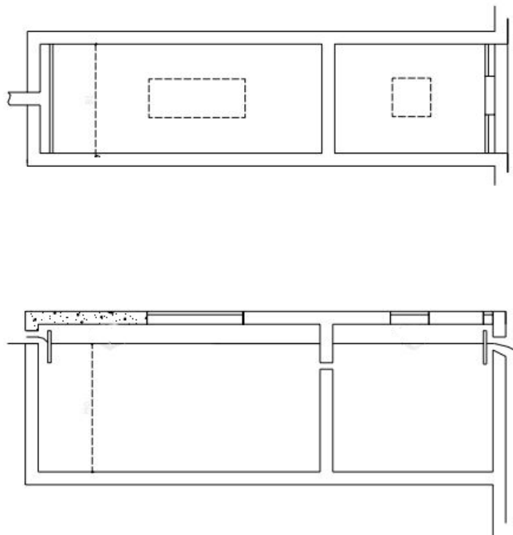
Σχήμα 2: Κάτοψη και τομή της σηπτικής δεξαμενής.
