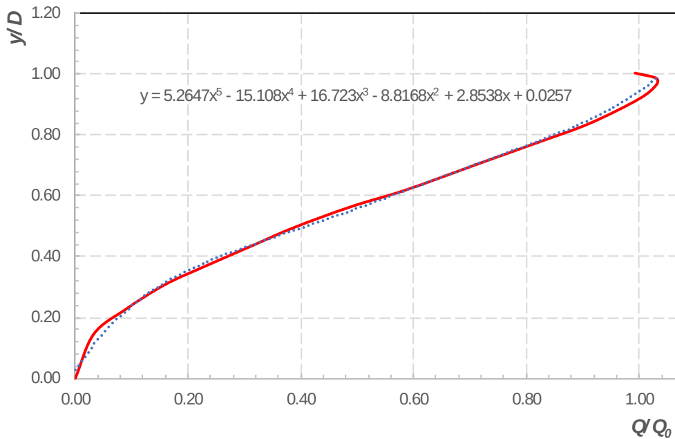
Σχήμα Π5: Πολυωνυμική σχέση παρεμβολής της μεταβολής των υδραυλικών μεγεθών ροής με ελεύθερη επιφάνεια σε κυκλικούς αγωγούς συναρτήσει του λόγου πλήρωσης y/D .
