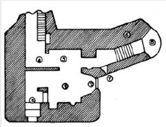
ΚΑΤΟΨΗ ΠΥΡΟΒΟΛΕΙΟΥ ΠΛΑΓΙΟΦΥΛΑΞΗΣ (Κλίμ. 1:150)
