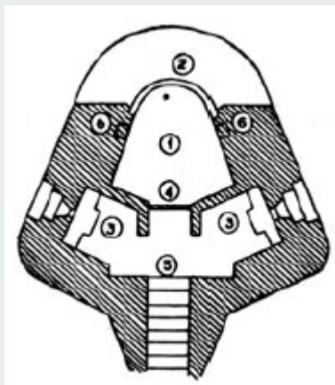
ΚΑΤΟΨΗ ΔΙΠΛΟ ΠΟΛΥΒΟΛΕΙΟ - ΠΑΡΑΤΗΡΗΤΗΡΙΟ (Κλίμ. 1:150)
